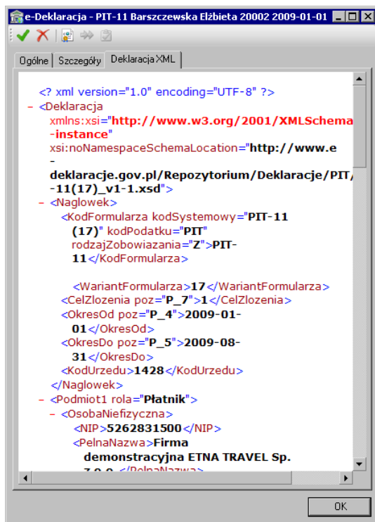
Rys. 14-46 Okno informacji o e-Deklaracji – panel Deklaracja XML .
