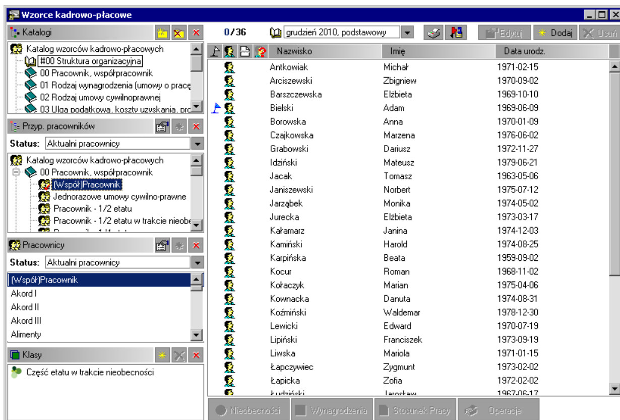
Rys. 5-4 Okno Wzorce .
