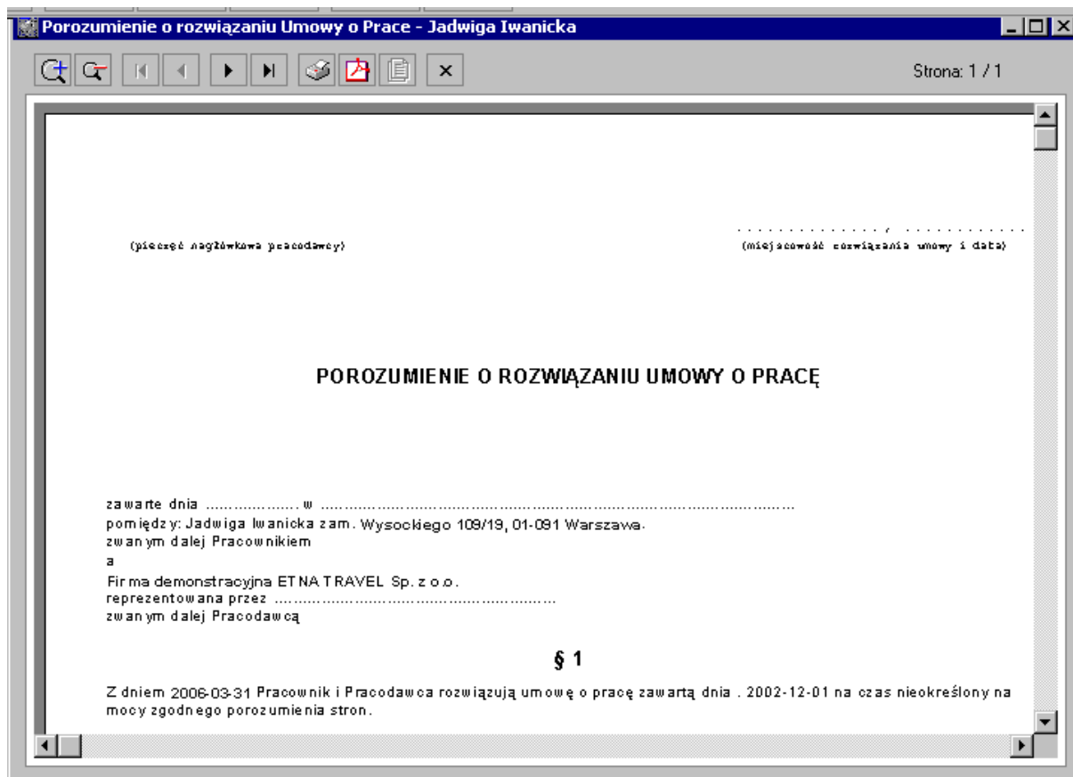
Rys. 4-57 Raport Porozumienie.
