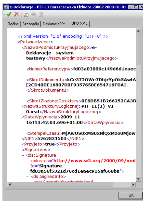
Rys. 14-50 Okno informacji o e-Deklaracji – panel UPO XML po potwierdzeniu e-Deklaracji i zwrocie UPO.
