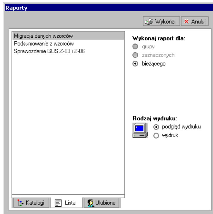
Rys. 14-10 Wybór raportu.
