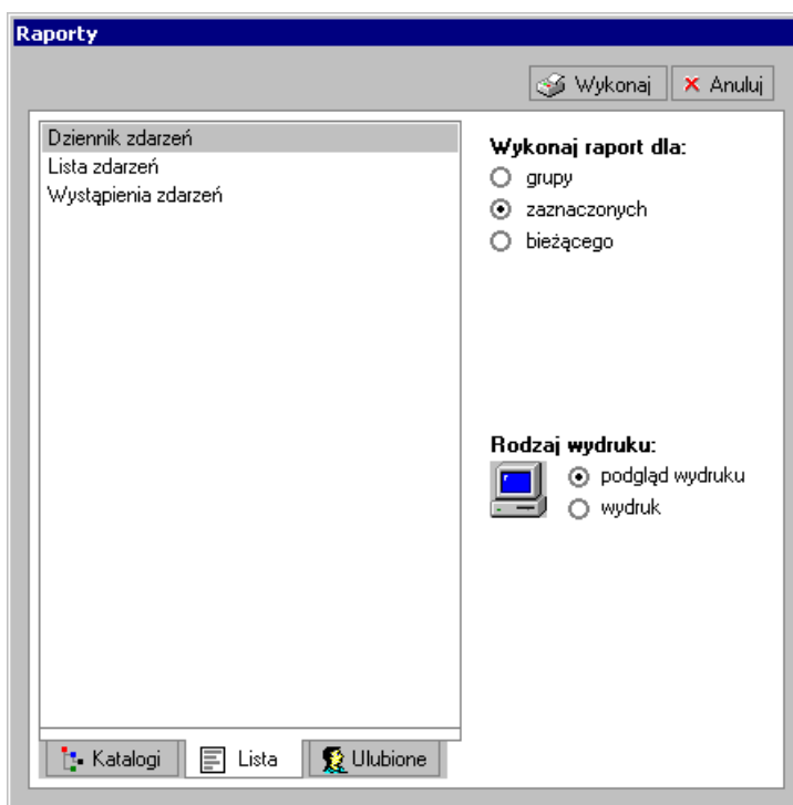
Rys. 14-21 Okno Raporty.
