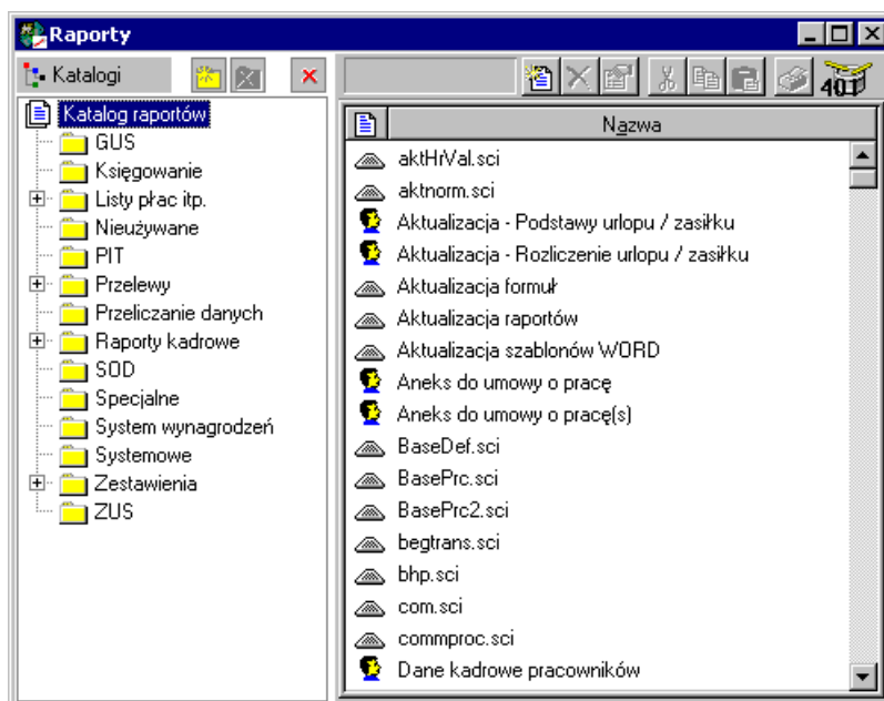
Rys. 14-52 Okno Raporty .
