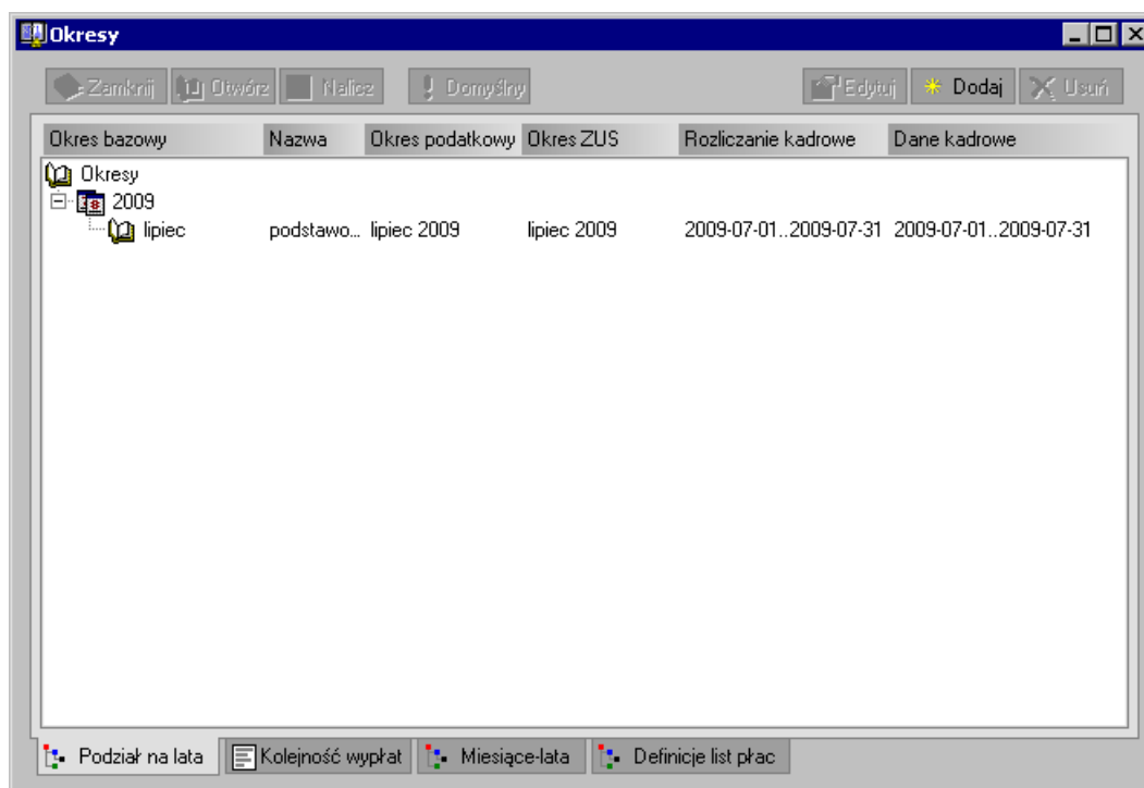
Rys. 4-4 Okno Okresy
