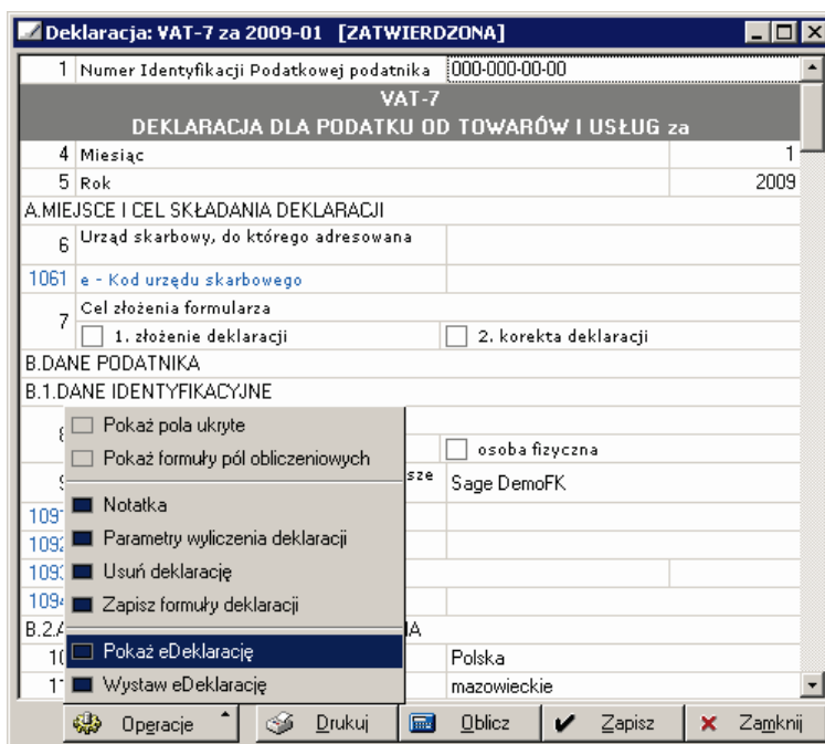
Rys. 10-17 Wywołanie okna o stanie e-deklaracji z programu Symfonia® Finanse i Księgowość
